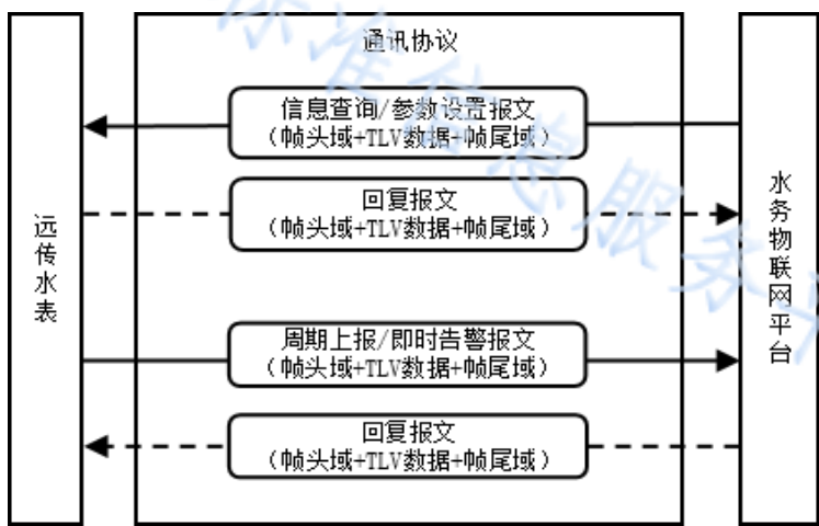
图1 通讯架构示意图
